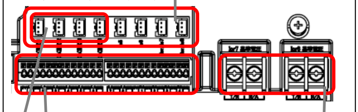
端子台・コネクタ拡大図
